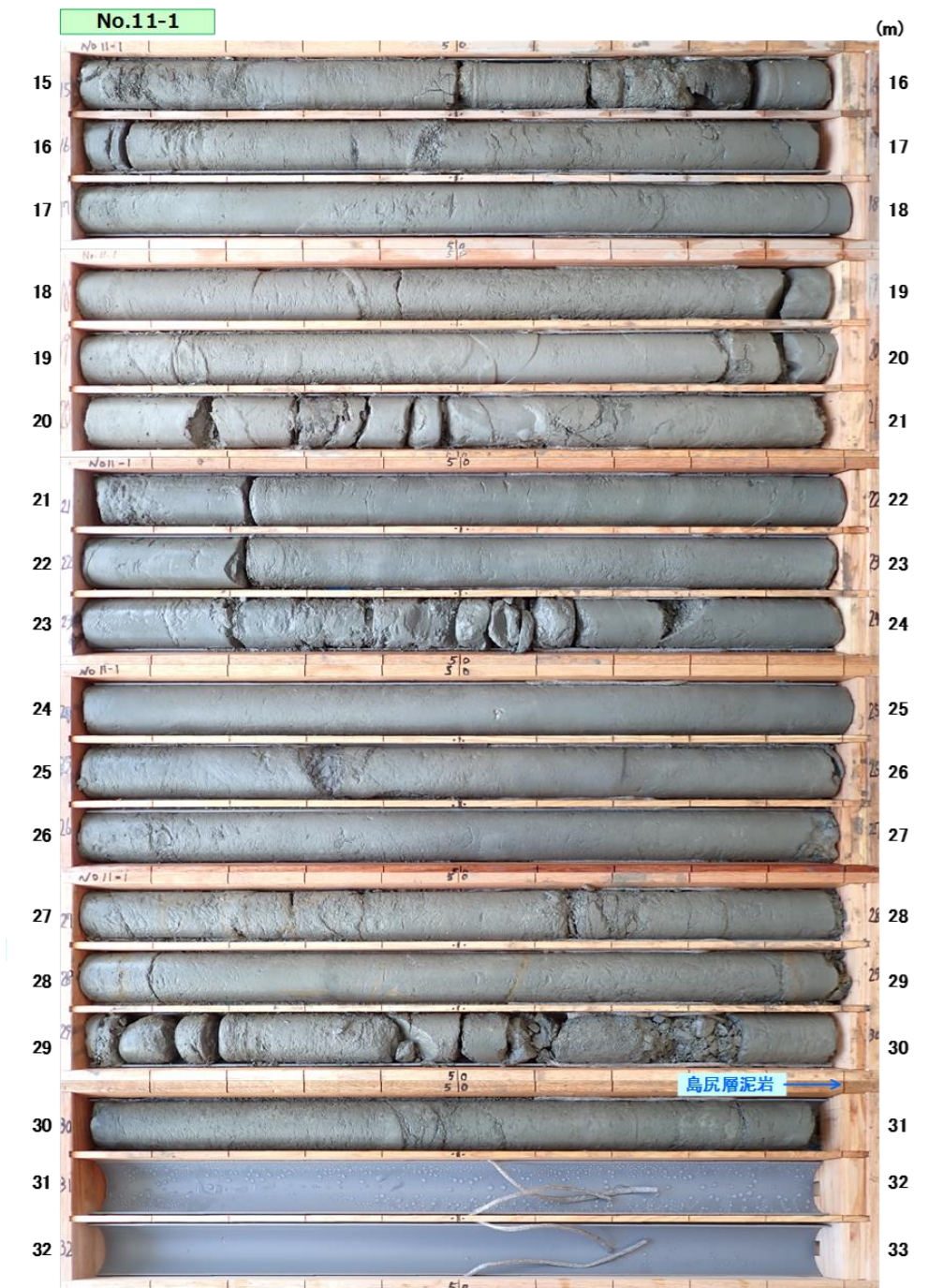
図 3.1.9(2) コア写真：No. 11-1
