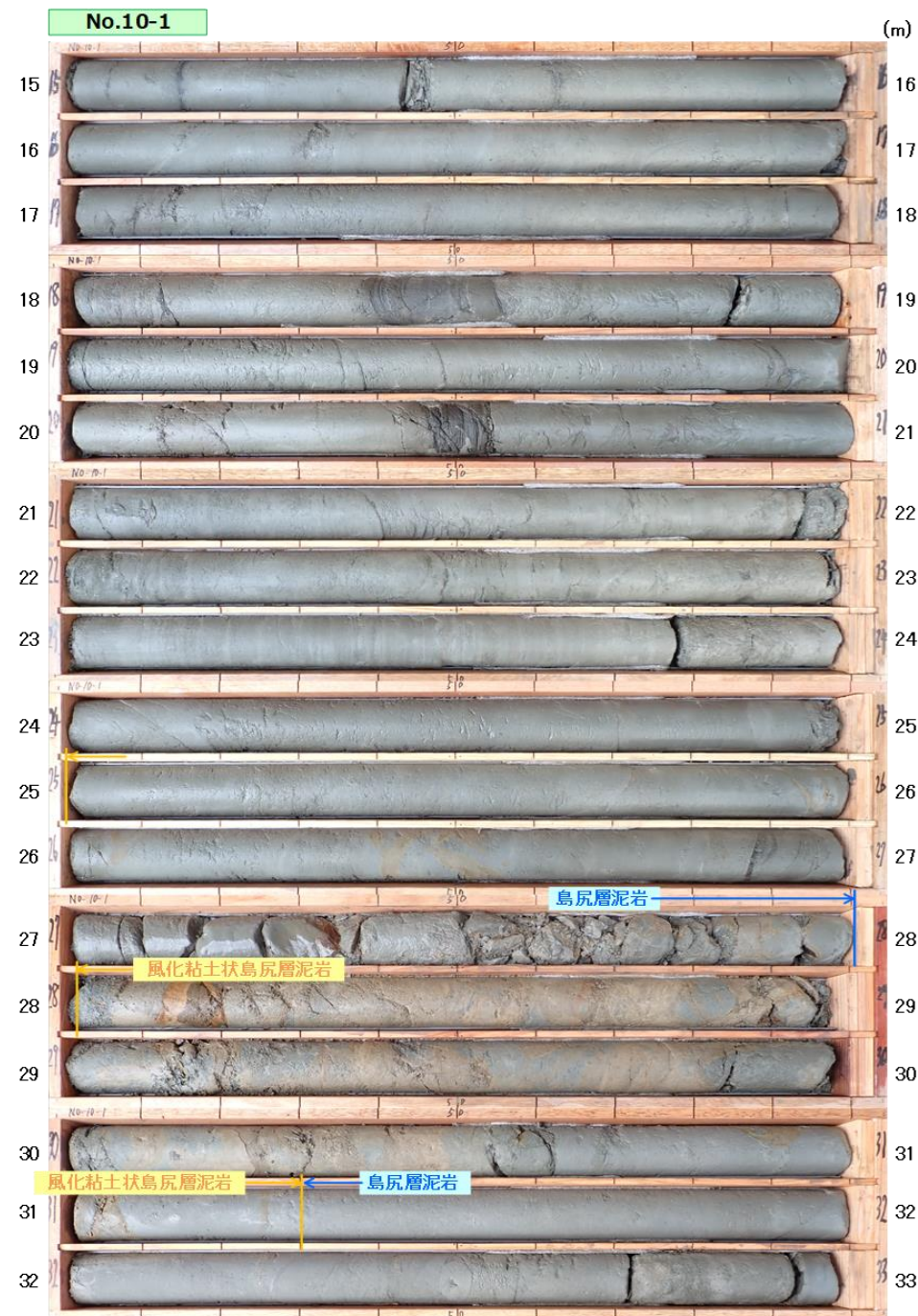
図 3.1.6(2) コア写真：No. 10-1
