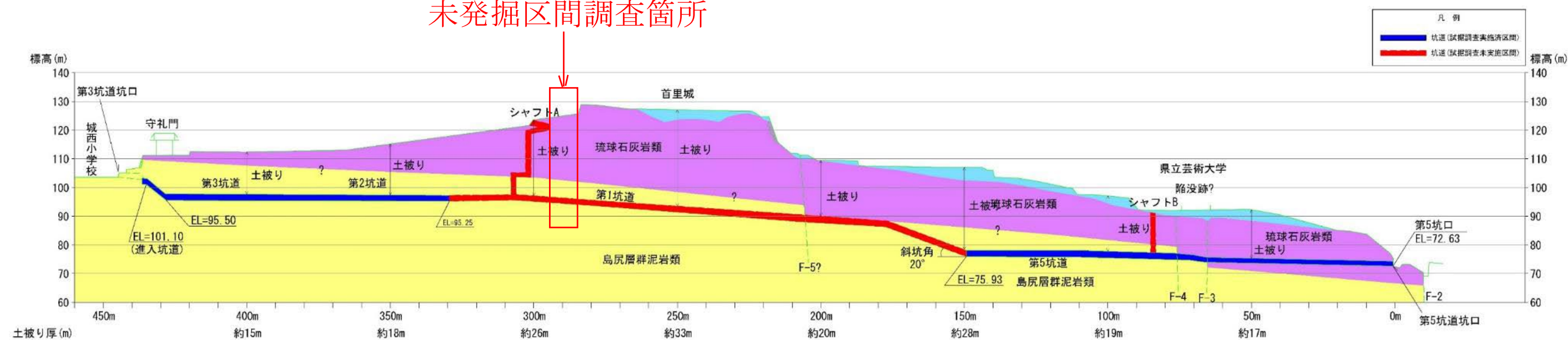
図 3.2.2 第32軍司令部壕周辺の地質平面図及び地質断面模式図
